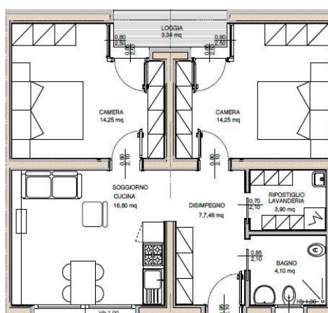
TIPOLOGIA A (TRILOCALE) (60 m 2 circa):
